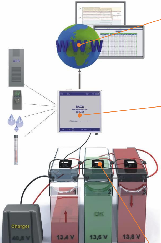
BACS® 网络管理系统 平衡第 1 与 3 颗电池的电压
