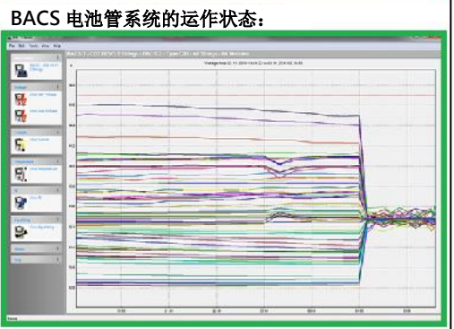
BACS® VIEWER 范例截图 图例上方是一个一般电池组已经运作达5年的各颗电池电压的分布曲线图，当启用 BACS® Equalization (Balancing) 专利技术的功能，可在下方图例看到，经过几个小时之后，各颗电池电压驱近一致，且合乎电池制造商的规范与电压差在 ± 0.01V 以内。
